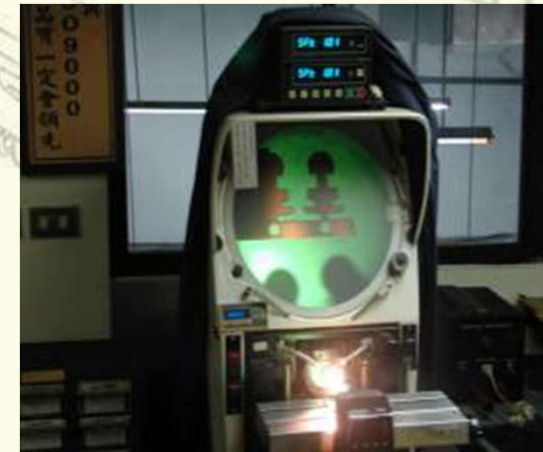
臥式投影機
