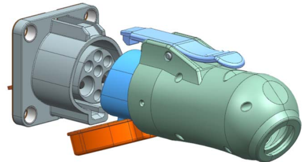
機車充電槍及充電座
